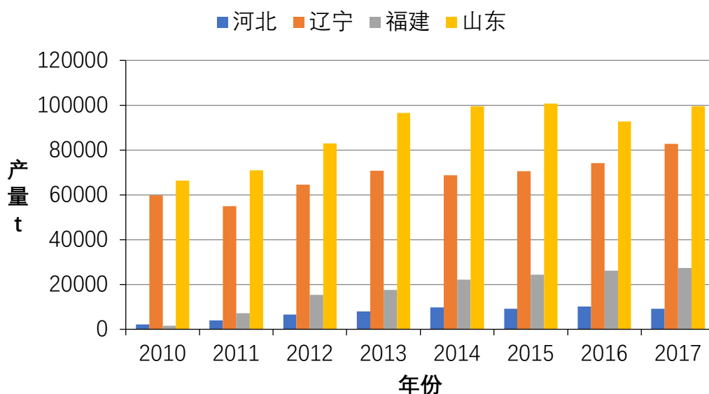
图 5 2010-2017 年中国海参海水养殖主要省份产量情况
